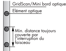
Figure 9.2 Effacement des faisceaux par pièce d'occultation
