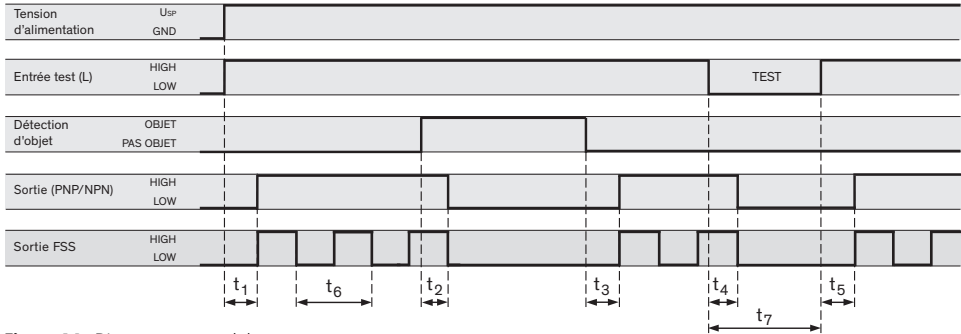
Figure 14: Diagramme général des temps
