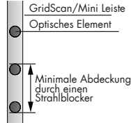
Abb. 9.2 Torausblendung durch Strahlblocker
